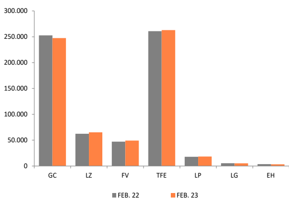
ENERGÍA ELÉCTRICA DISPONIBLE SEGÚN ISLAS (Mwh) FEB. 22-23
