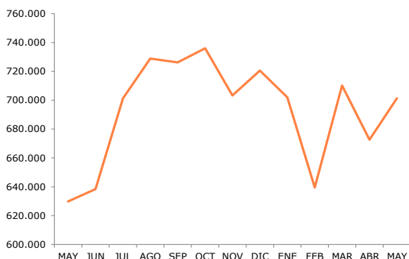
ENERGÍA ELÉCTRICA DISPONIBLE. CANARIAS (Mwh) MAY. 21-22
